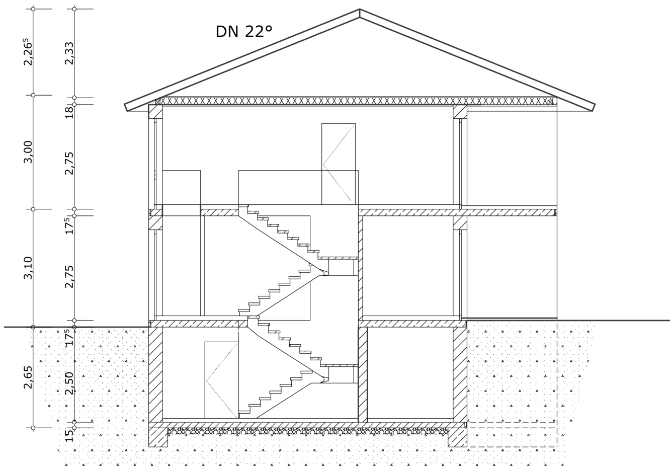
Schnitt 01
