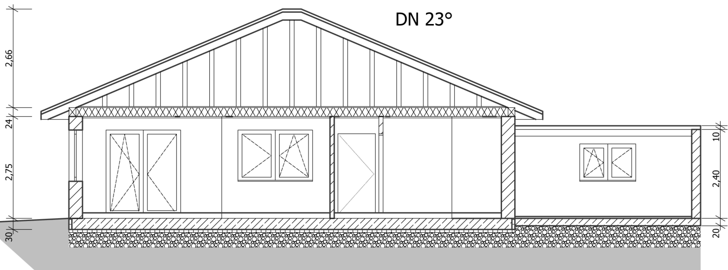
Schnitt 02
