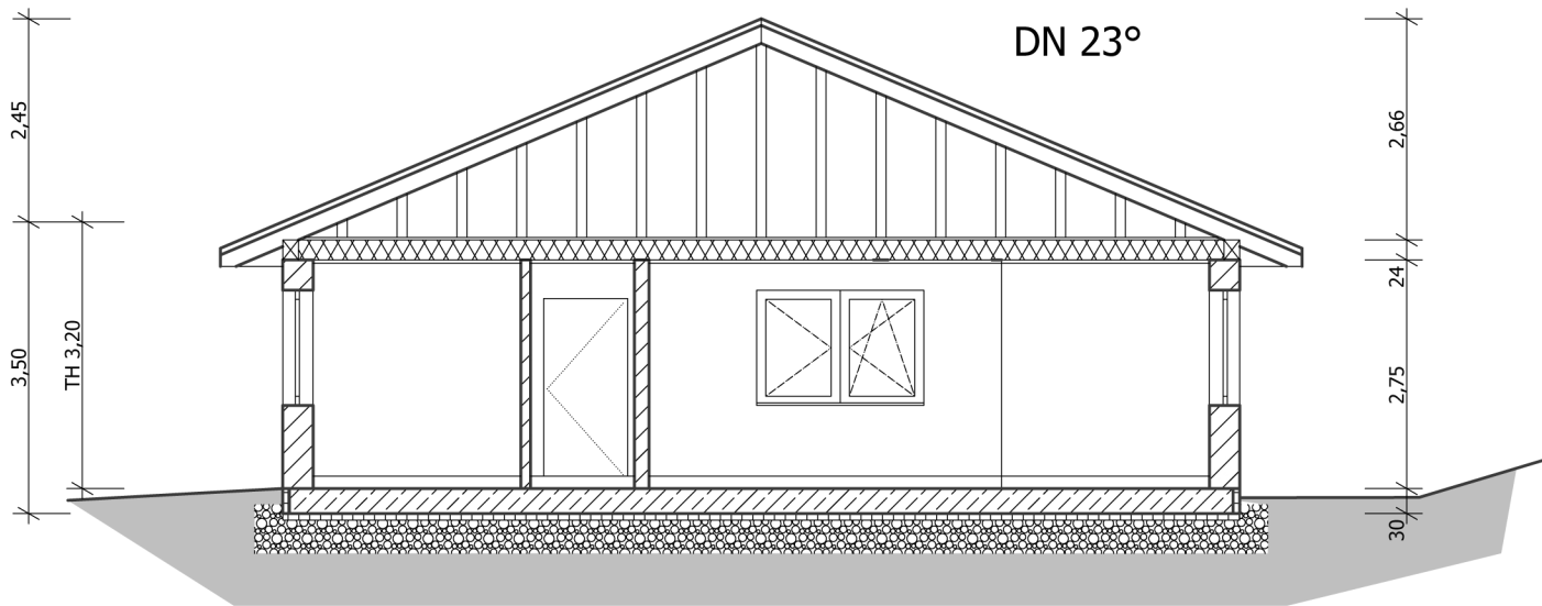
Schnitt 01
